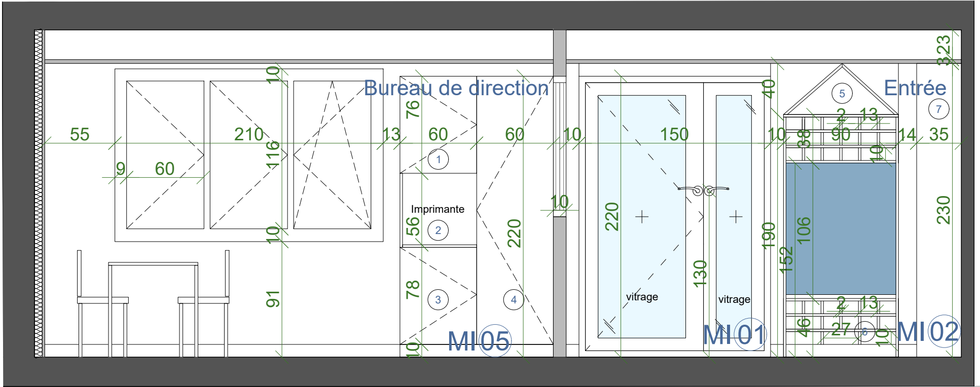
COUPE AA'
