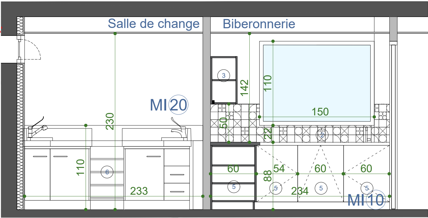
COUPE BB'
