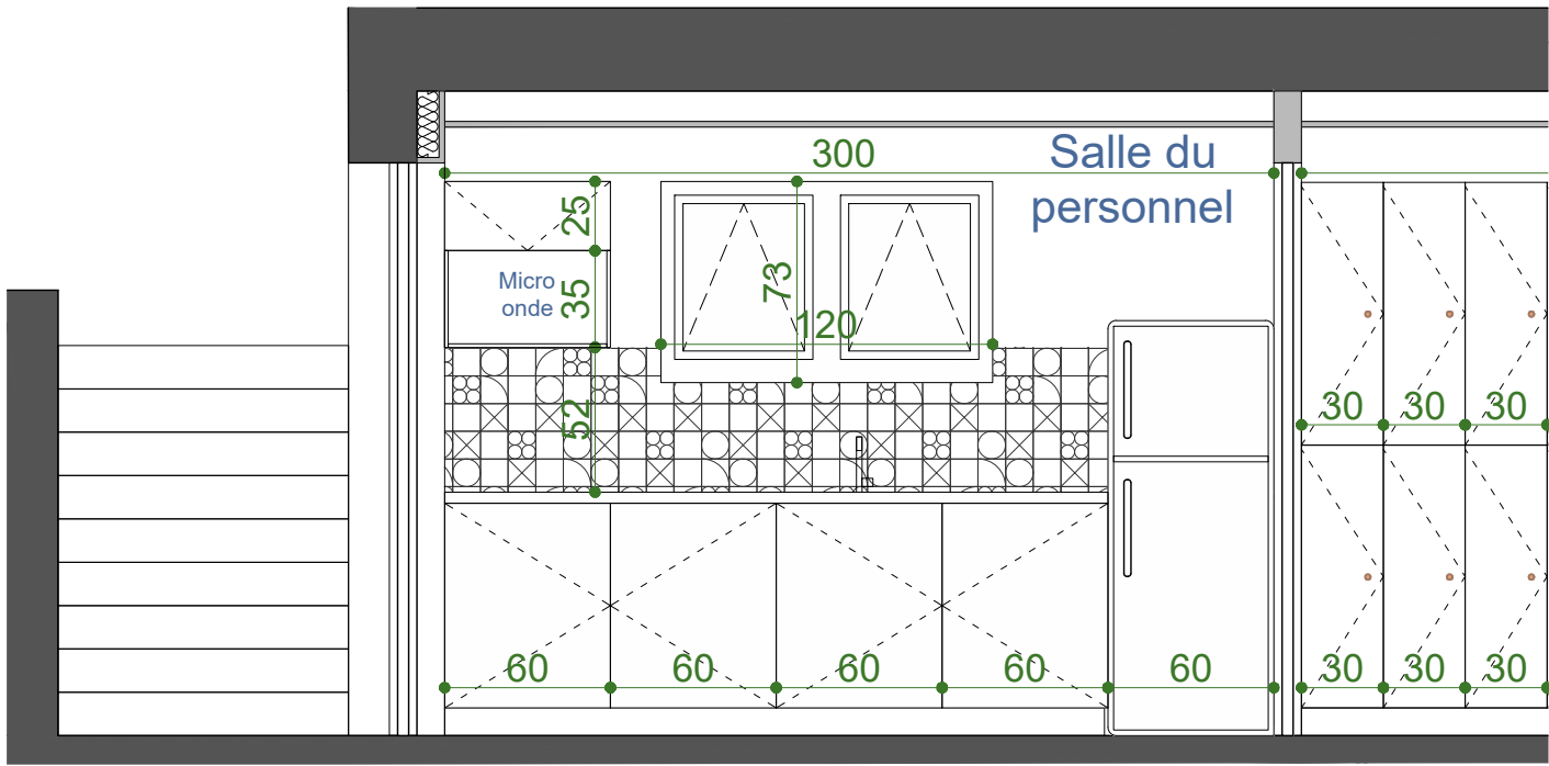
COUPE AA'
