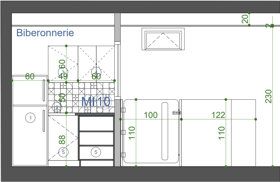
COUPE AA'
