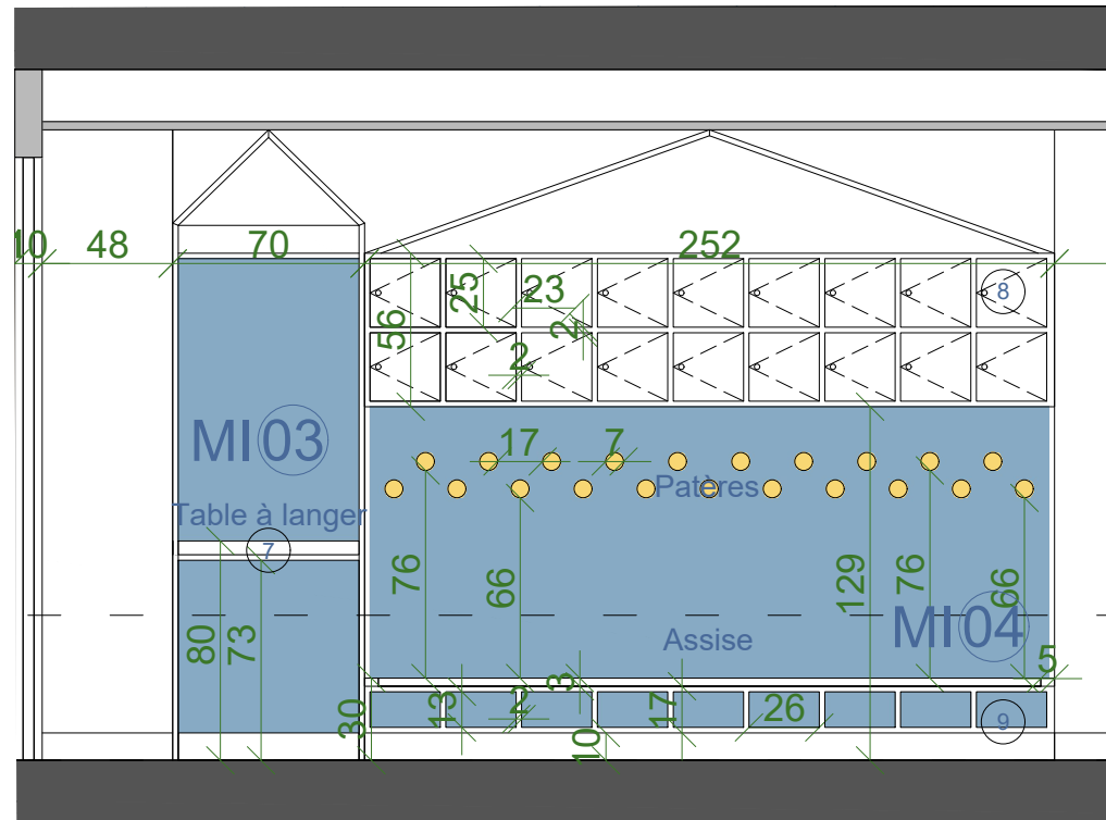
COUPE CC'
