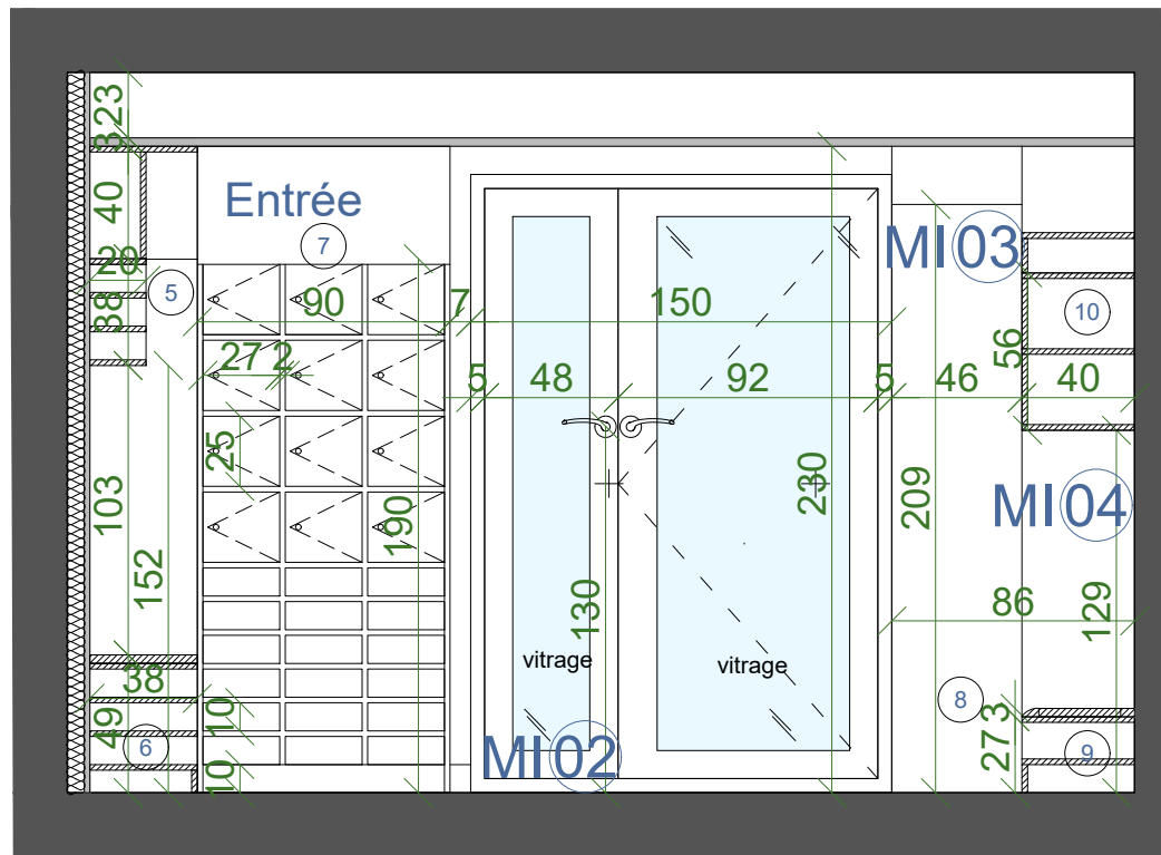
COUPE BB'
